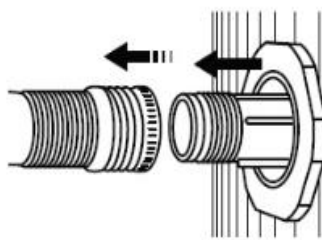
6. Nehmen Sie nach erfolgter Entleerung (in geschlossener, vollständig herausgezogener Position) den Schlauch ab und bringen Sie die Verschlusskappe wieder an
