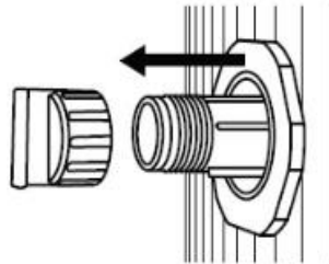
2. Stülpen Sie das geschlossene Ventil vollständig heraus, nehmen Sie die Kappe ab und bewahren Sie diese sicher auf
