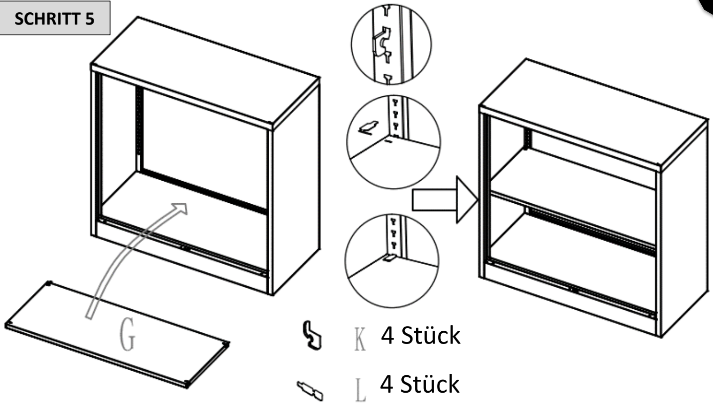
5. Setzen Sie den Zwischenboden G ein
