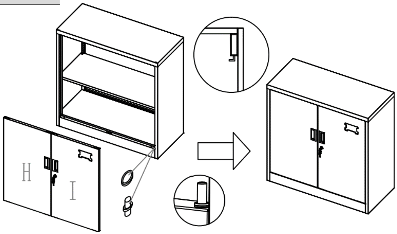
6. Bauen Sie die Türen H und I ein
